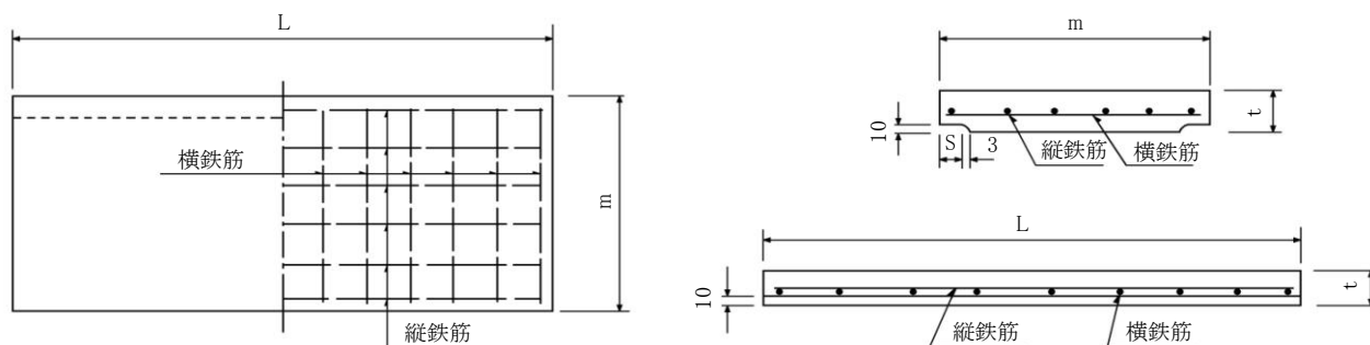
■ I 型の寸法及び配筋表 t - 14
