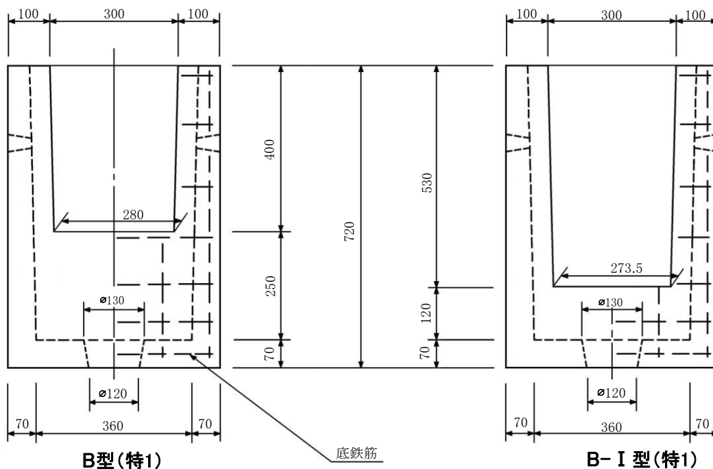
〔開口部寸法〕
