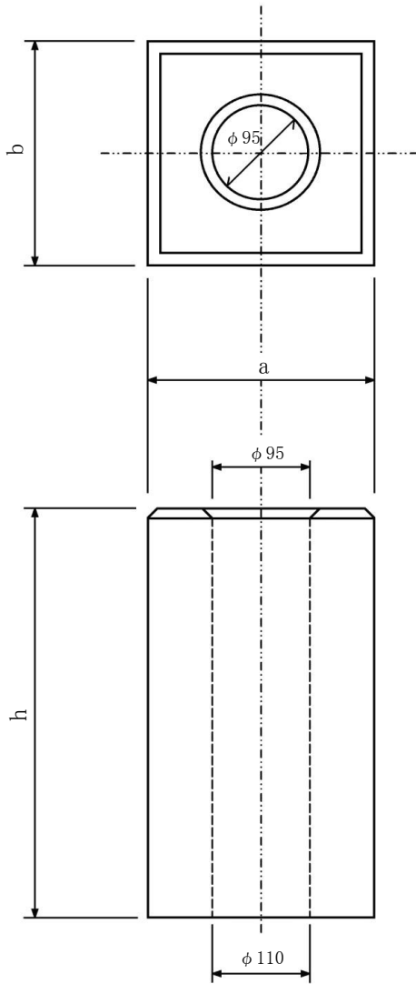
呼び 180□タイプ
