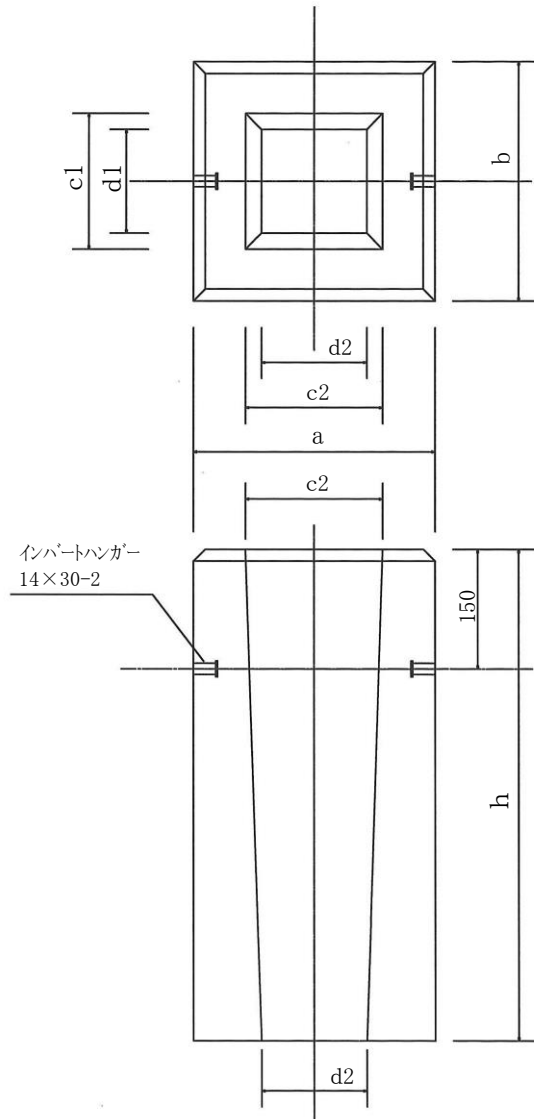
呼び 300□タイプ
